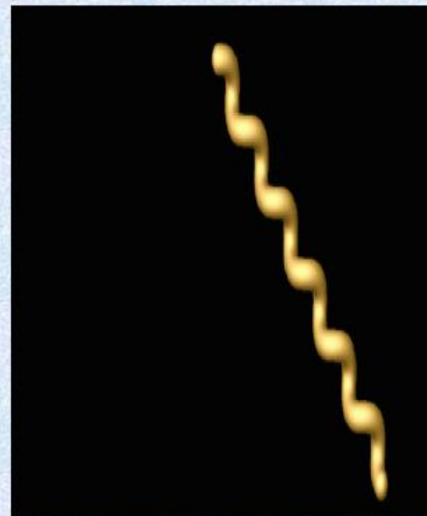
Motilitas spiroplasma
